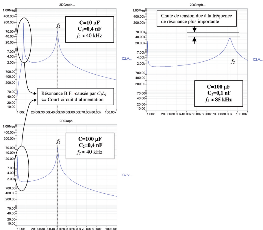
Figure 9 : Simulations sous Simploter [4].
