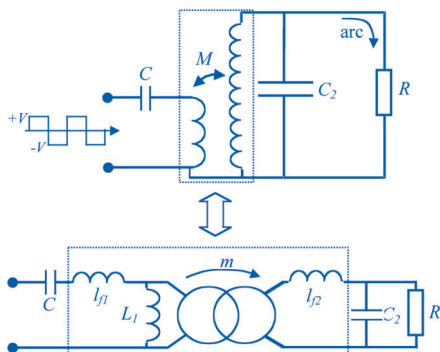
Figure 6 : Modélisation du transformateur équivalent.
